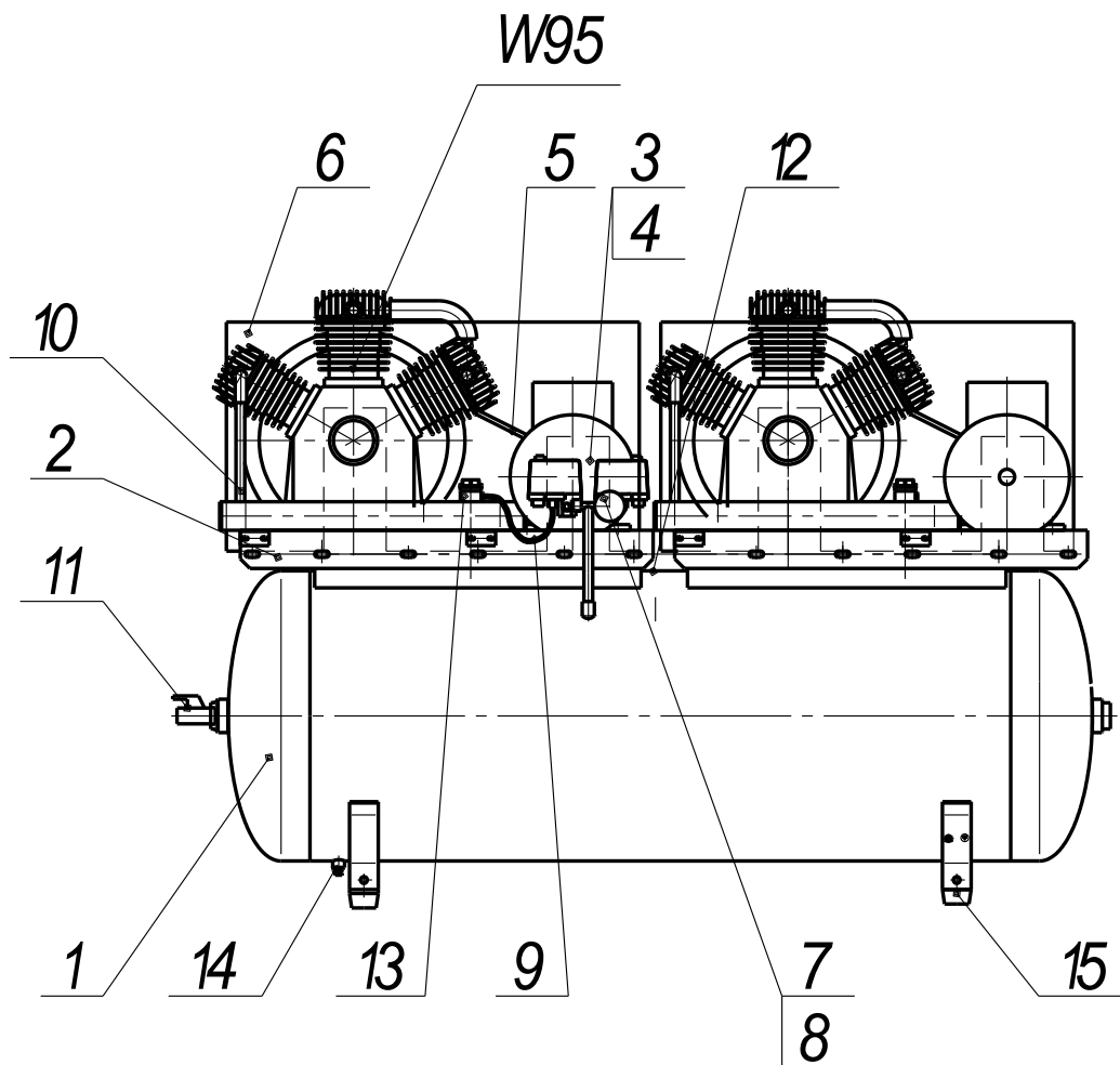
Рисунок 4 – Общий вид компрессора СБ4/Φ-500.W95ТБ
