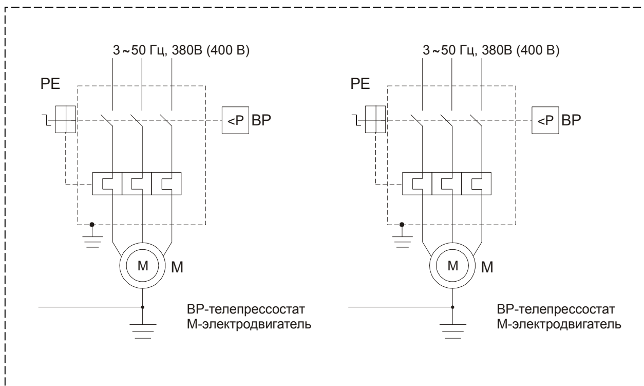
Рисунок 5 – Схема электрическая принципиальная СБ4/Φ-500.W95ТБ
