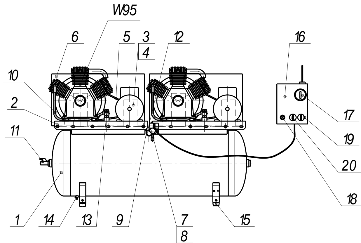
Рисунок 1 – Общий вид компрессора СБ4/Φ-500.W95Т
